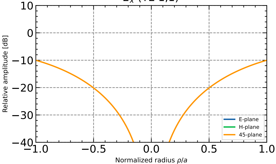
E_x (TE 1,1)
