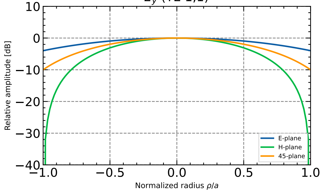
E_y (TE 1,1)
