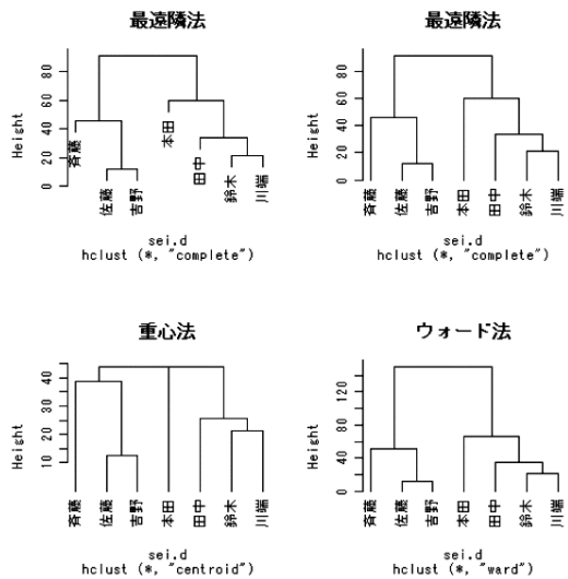
図 4 ユークリッド距離の樹形図
