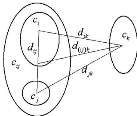
図3 クラスター間の距離
