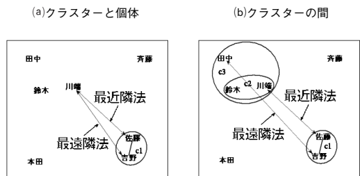
図2 コーフェン距離
