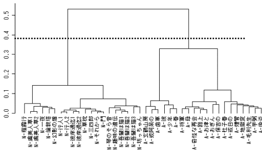
図1 芥川と夏目の作品の樹形図
