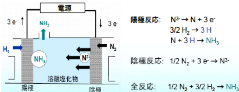
常圧アンモニア電解合成の原理
