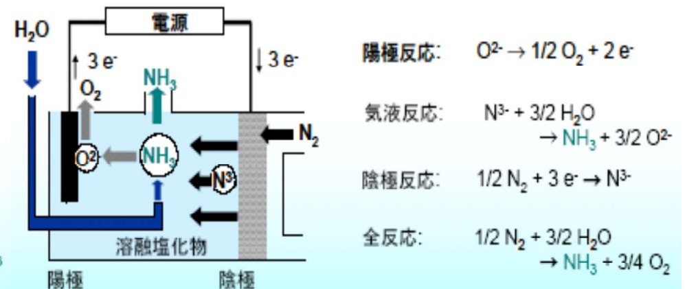
窒素と水からの常圧アンモニア電解合成
